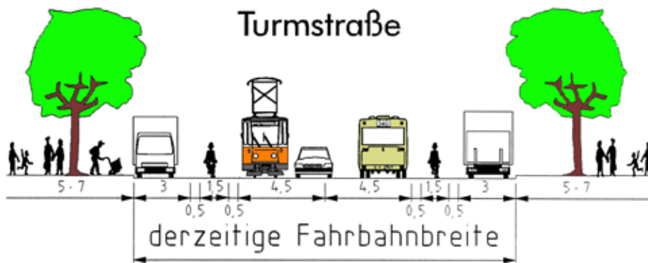
Mögliche Fahrbahnaufteilung in der östlichen Turmstraße, hier mit inzwischen historischen Fahrzeugen. Es wären auch andere Varianten möglich, z.B. der Erhalt der Gehölze auf dem Mittelstreifen unter Verzicht auf die Überholmöglichkeit, oder eine Fußgängerzone mit Zufahrt nur für Straßenbahn/Bus, Radfahrer und Lieferverkehr.
